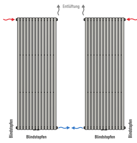
Seitenanschluss
