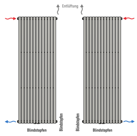
Seitenanschluss
